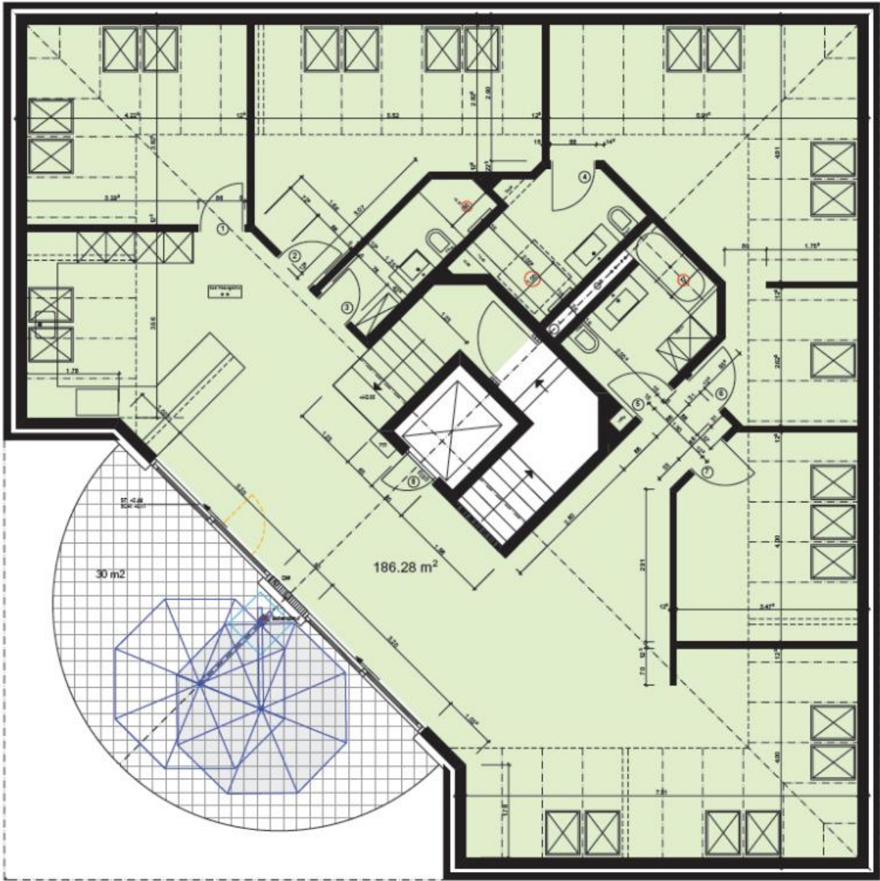
Grundrissplan 5.5 Zimmer-Dachgeschosswohnung, Gladbachstrasse 95, 8044 Zürich
